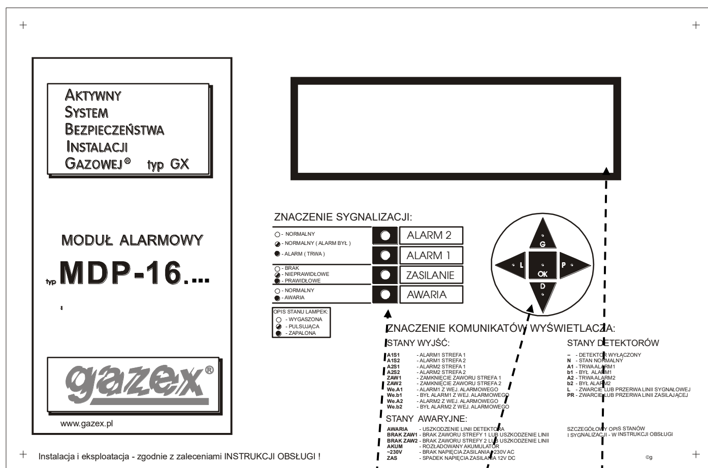
Rys.2.1. Widok płyty czołowej (pod pokrywą przeźroczystą)
