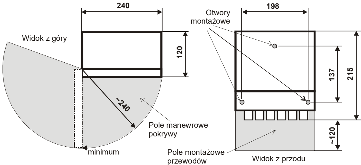
Rys.3. Wymiary podano w [mm]. Szablon wierceń pod otwory montażowe MD wydrukowano na opakowaniu tekturowym.
