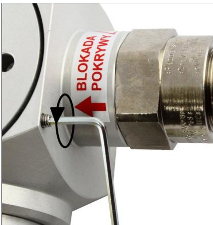
Rys.3.3. PRZED odkręcaniem pokrywy ==> odkręcić wkręt BLOKADY POKRYWY:
